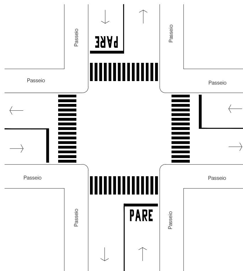
Planta Baixa - Detalhe dos Cruzamentos Conforme Resolução nº 236 - CONTRAN S/Escala
