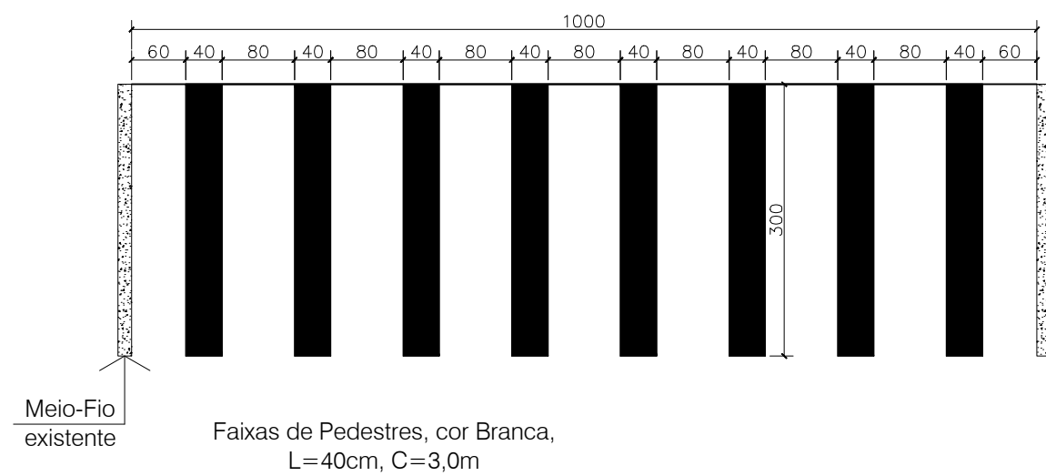
Planta Baixa Faixa de Pedestres, conforme Resolução nº 236 - CONTRAN S/Escala
