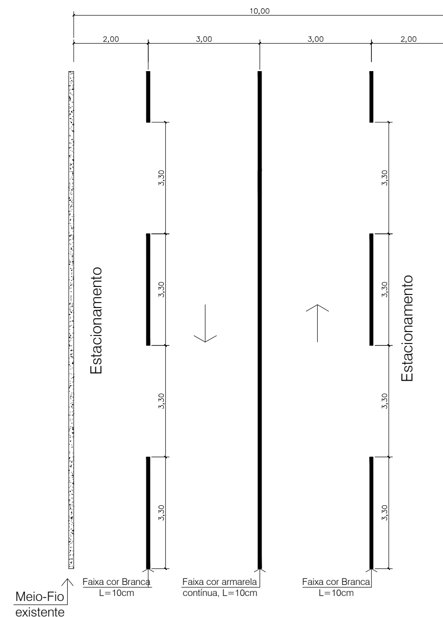
Planta Baixa Faixas nas Vias, conforme Resolução nº 236 - CONTRAN S/Escala
